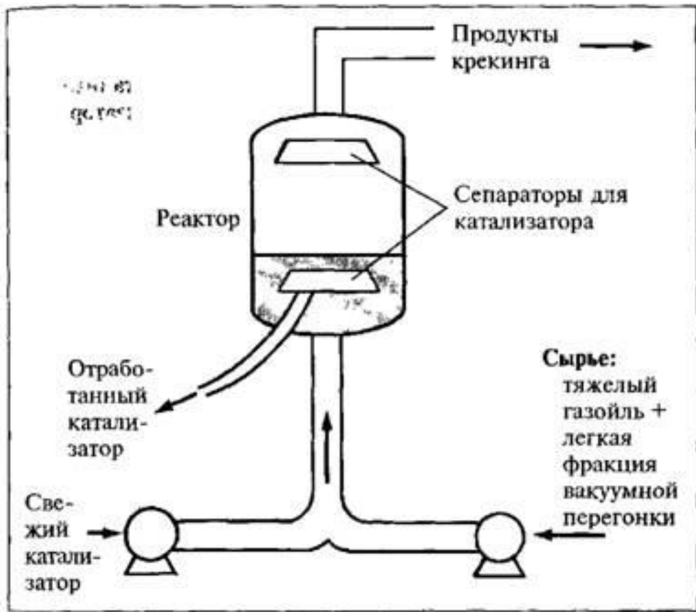
Рис. 6.1. Реакторный блок каталитического крекинга.
